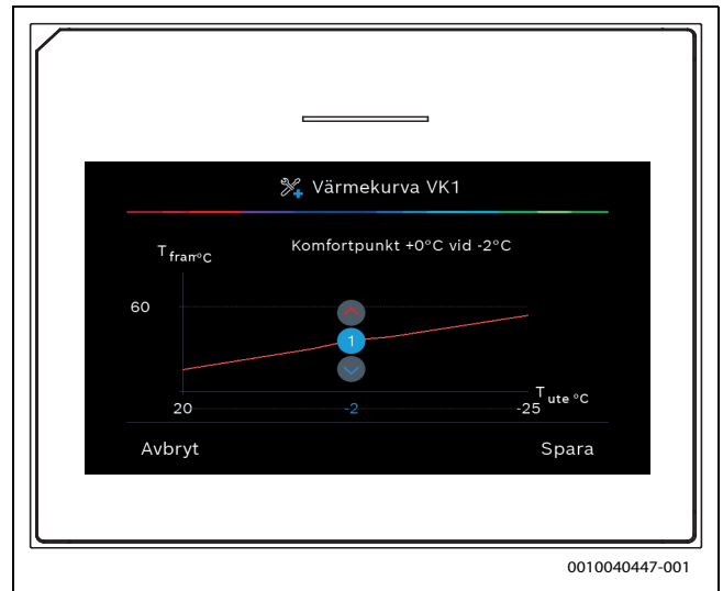
Bild 11 Justera komfortpunkt (böjning av värmekurva), vid inställning med extra baspunkt
