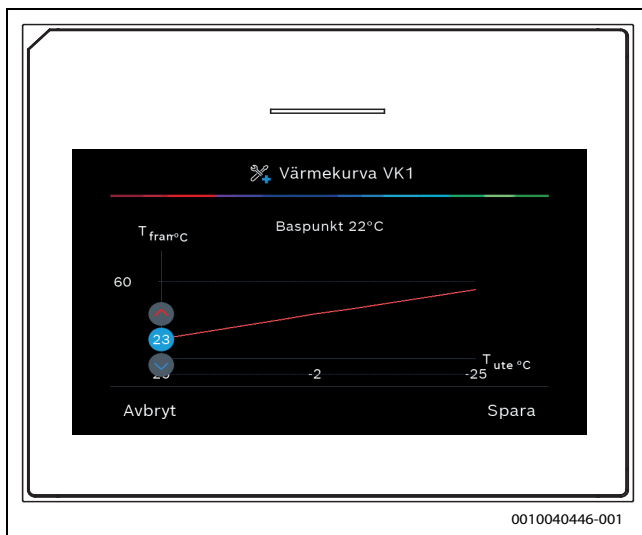
Bild 10 Justera baspunkt vid inställning med extra komfortpunkt
