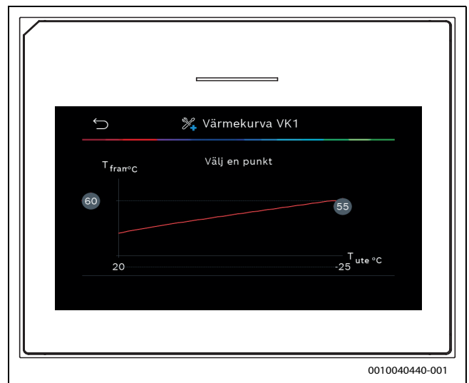
Bild 12 Utgångsvisning värmekurva vid inställning med endast ändpunkter
