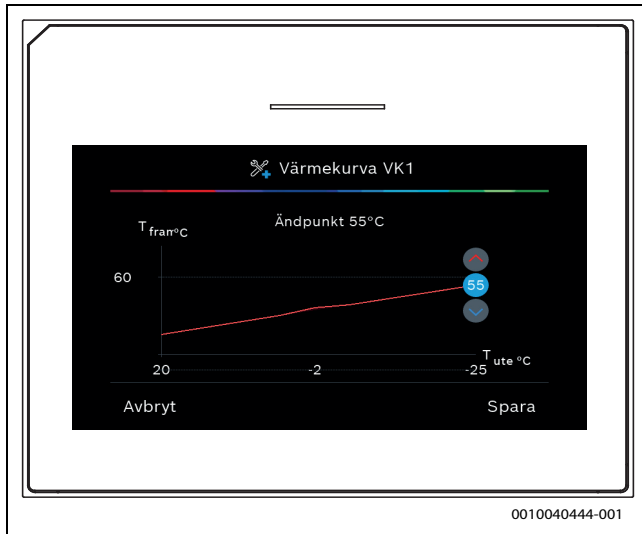
Bild 9 Justera ändpunkt vid inställning med extra komfortpunkt
