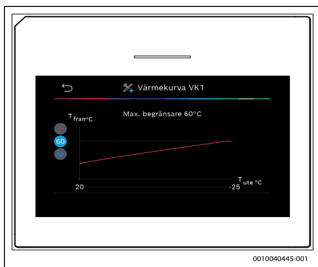
Bild 14 Justera maximal framledningstemperatur vid inställning med enbart ändpunkter
