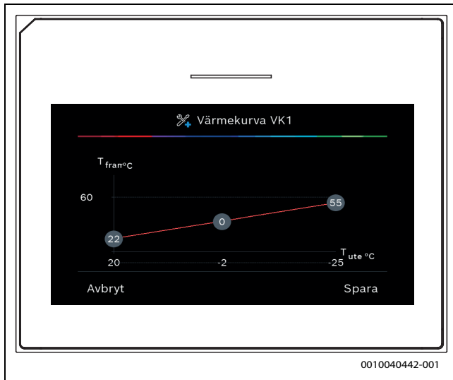
Bild 8 Utgångsvisning värmekurva vid inställning med extra komfortpunkt
