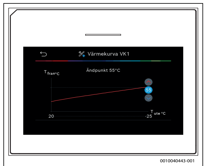
Bild 13 Justera ändpunkt vid inställning med endast ändpunkter
