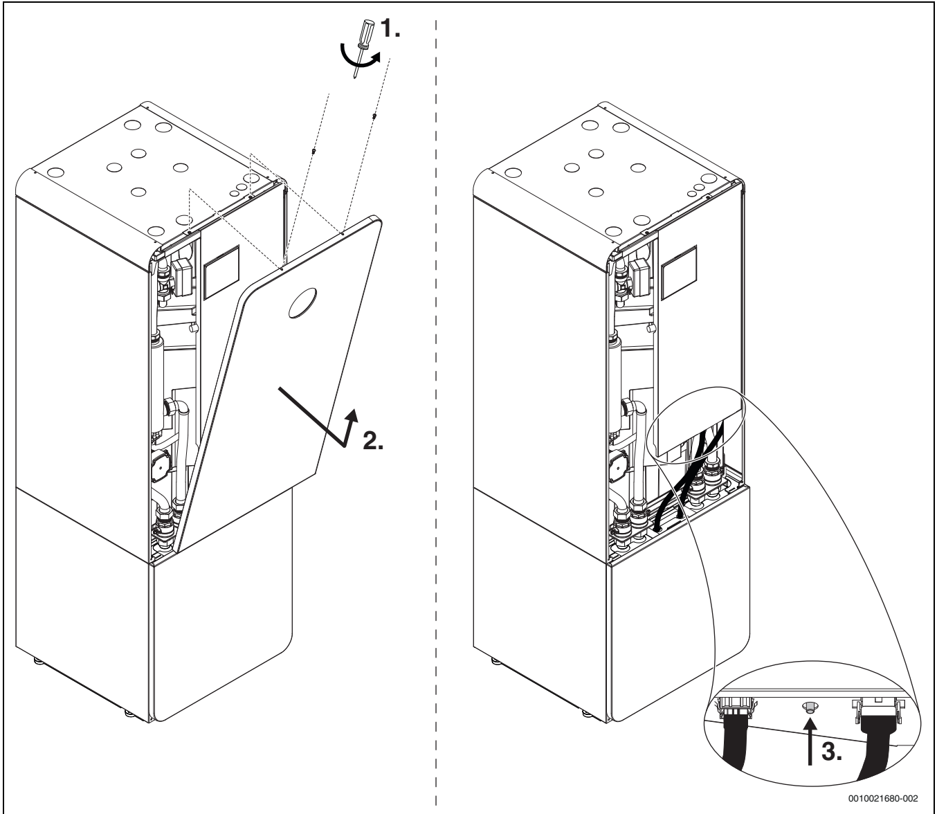
Bild 16 Återställning överhettningsskydd
